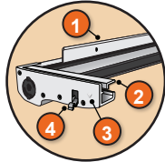
Carcasa de la malla
